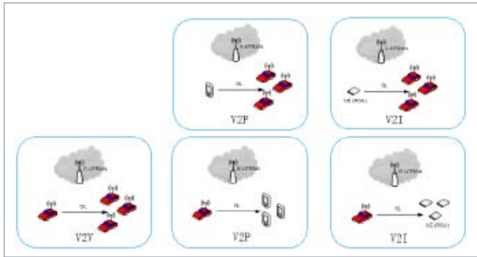
图13 LTE-V2X通信应用场景1-仅PC5接口
