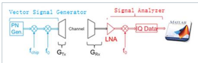
图4 时域信道测量框图
