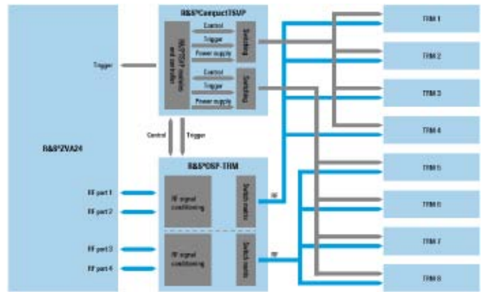
图19 系统扩展框图
