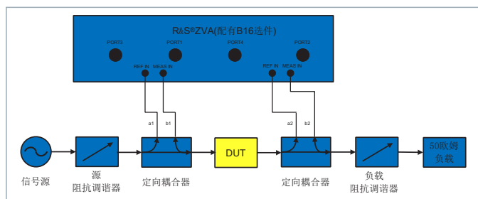
图6 矢量接收机负载牵引测量系统
