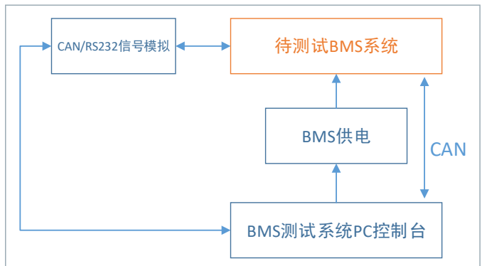
图11 系统间通信功能测试
