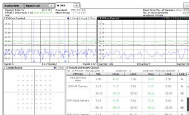
图31 DSRC/IEEE 802.11p EVM测试
