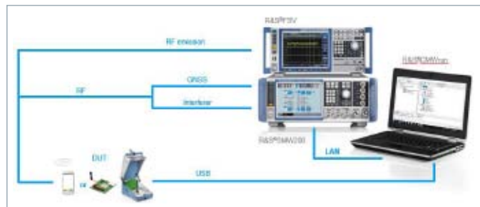
图61 车载导航RED测试框图
