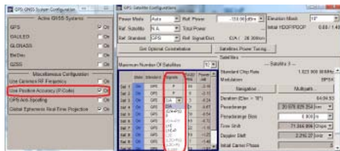
图26 GPS P码测试设置
