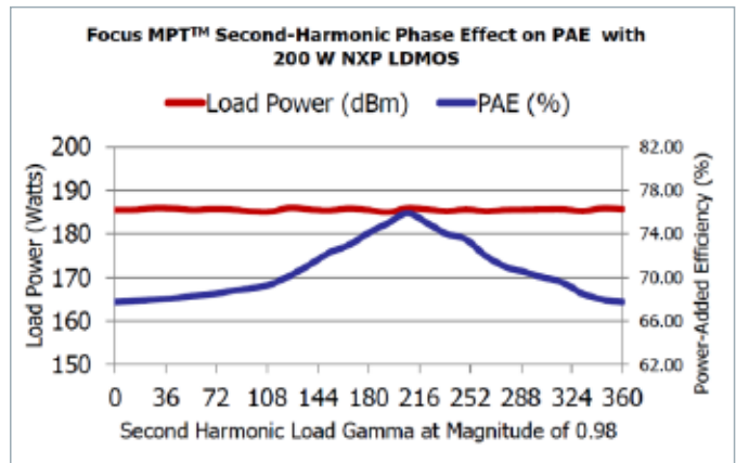
图3 二次谐波处的阻抗相位对PAE的影响。
