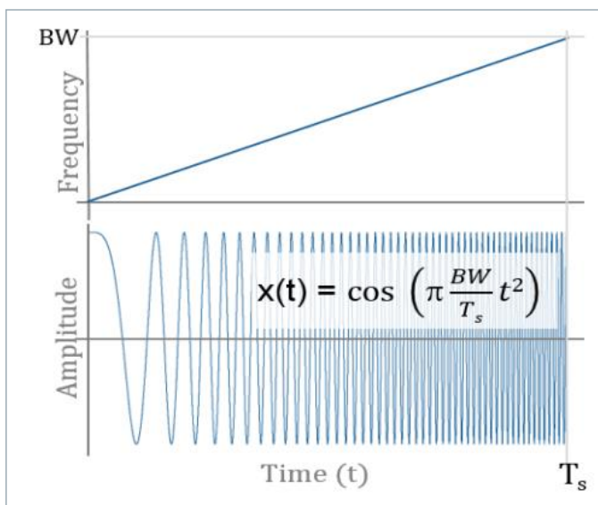
图1 一个线性调频脉冲内上升斜率信号示意
