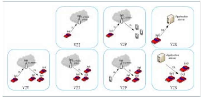
图14 LTE-V2X通信应用场景2-仅Uu接口
