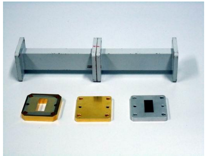
图7 波导传输/反射法测量夹具及校准件
