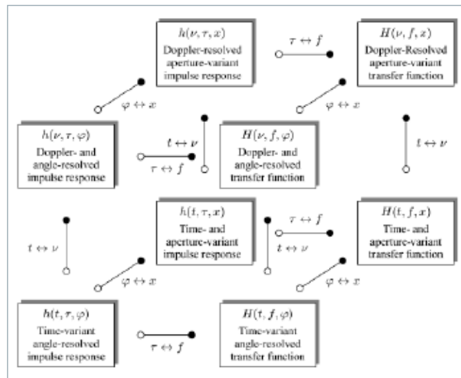
图1 信道系统函数
