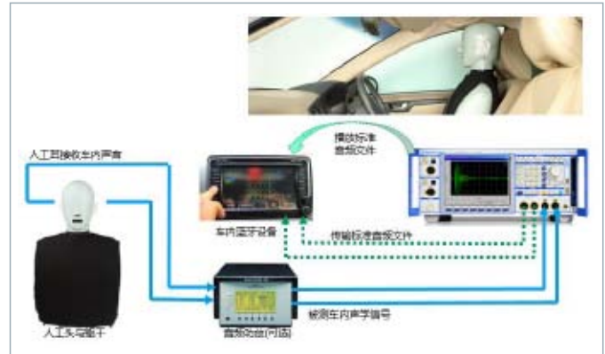
图67 车内蓝牙语音质量评估框图
