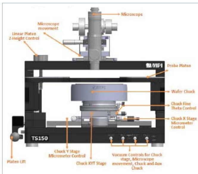
b 主机台主要部件 图2主机台
