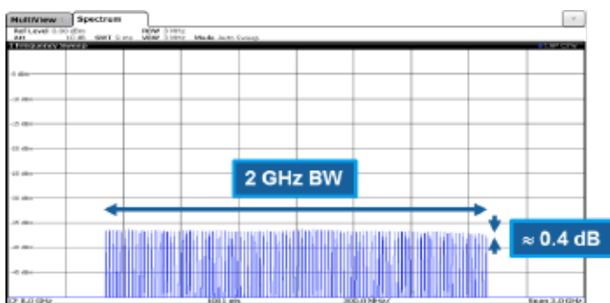
SMW200A 2 GHz宽带多音信号幅度平坦度测试图
