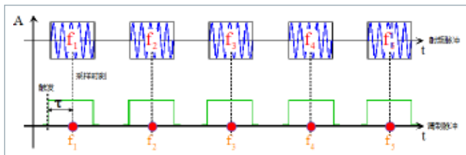
图7 ZVA采用脉内取点法测试脉冲S参数
