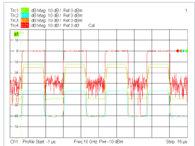
图9 ZVA脉冲时域参数测试的时域包络数据
