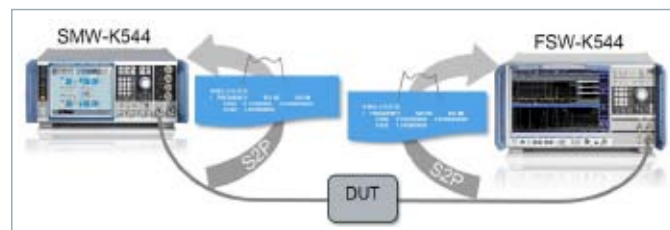
信号源和频谱仪外部频响实时修正方法示意图
