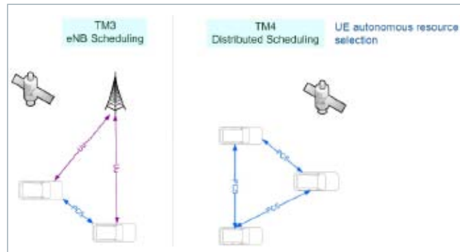
图19 LTE-V2V两种传输模式
