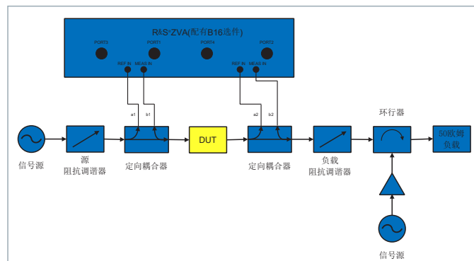
图7 混合型负载牵引测量系统
