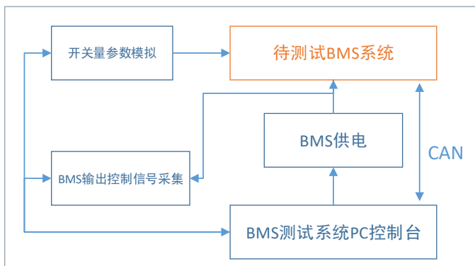
图13 开关量参数模拟测试
