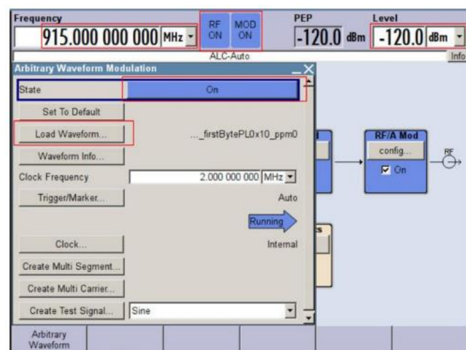
图10 矢量信号源设置界面
