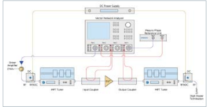
图4 Cardiff Model Plus测量系统
