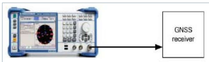
图12 导航接收机传导测试
