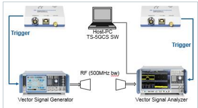
图6 绝对时延信道测量方案
