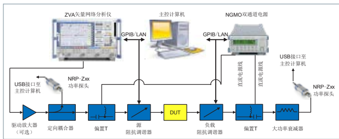
图3 基于ZVA矢量网络分析仪的负载牵引测量系统
