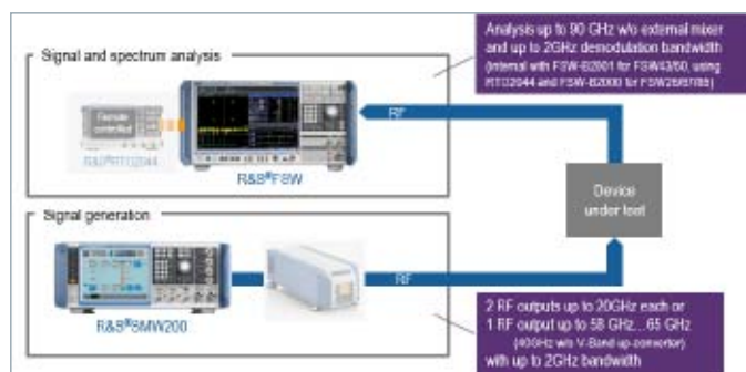
图53 5G URLLC测试方案
