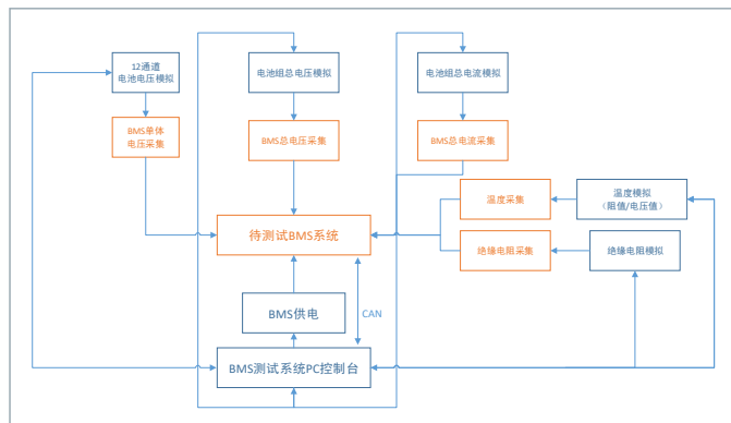
图9 BMS系统过压和欠压运行测试
