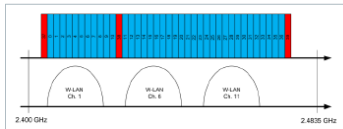
图1：蓝牙低功耗的信道分布
