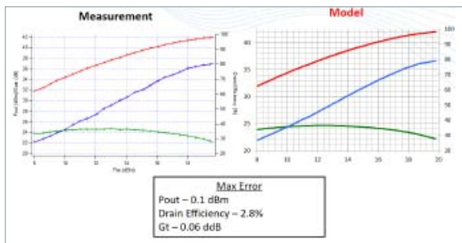
图7 Cardiff Model Plus模型仿真结果与实测结果比较
