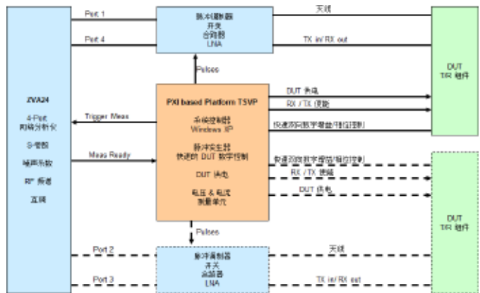
图2 TRM综合测试系统原理框图
