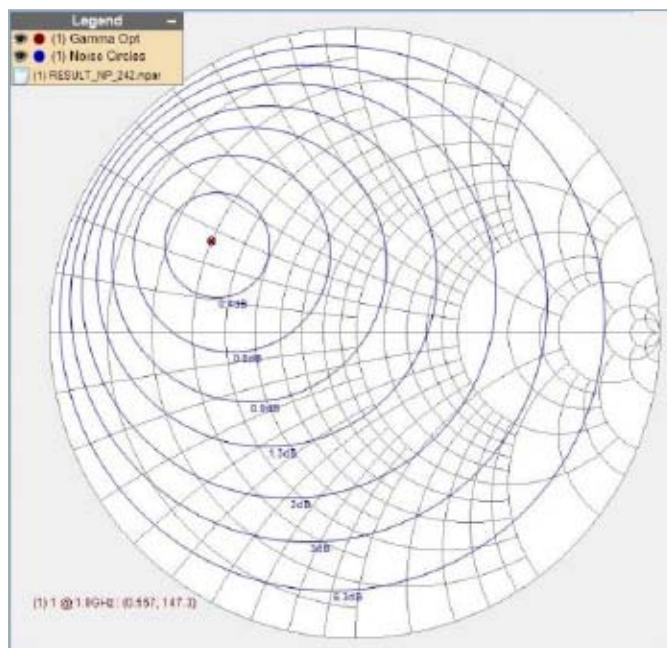
图2 噪声参数
