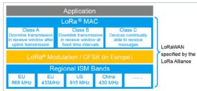
图3 LoRaWAN协议栈
