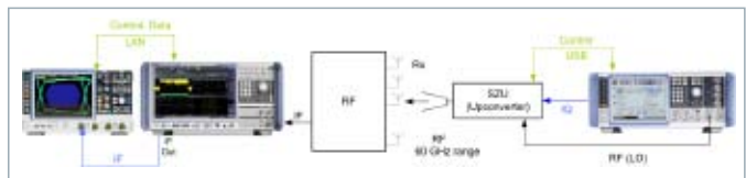
图12 RFIC的RX部分测试框图
