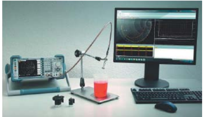
图11 同轴探针法测量系统
