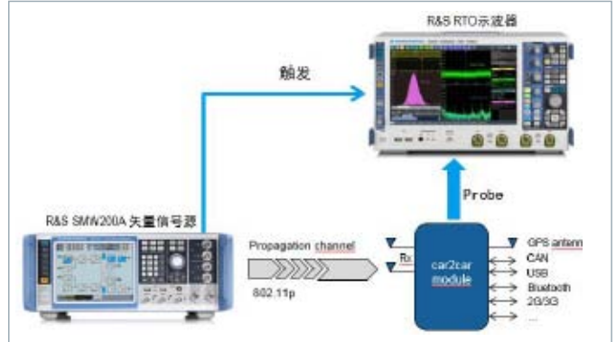
图37 DSRC/IEEE 802.11p空闲信道评估测试框图
