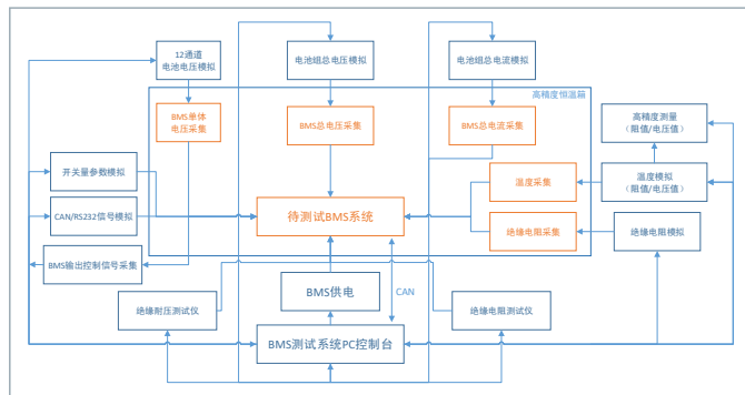
图2 BMS测试系统框图
