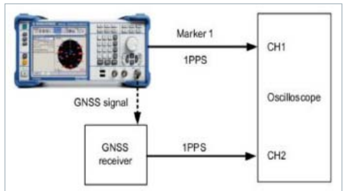
图23 接收机秒脉冲测试框图
