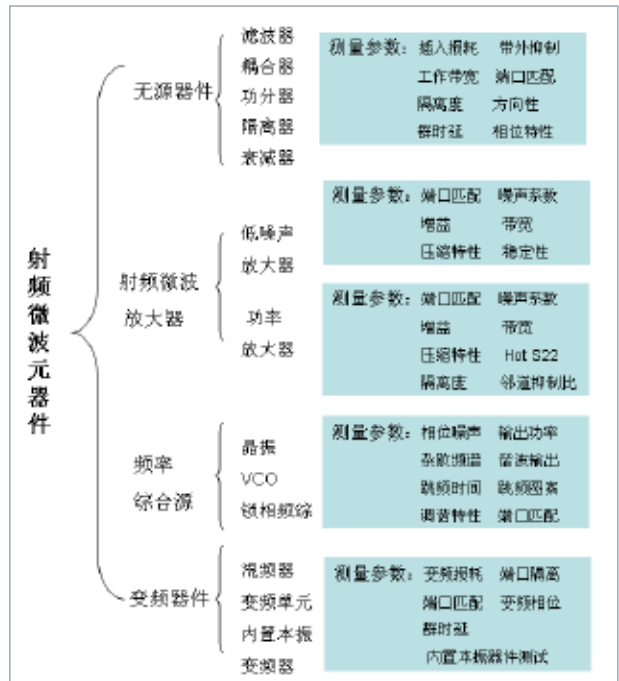
图1：元器件测试类型与指标
