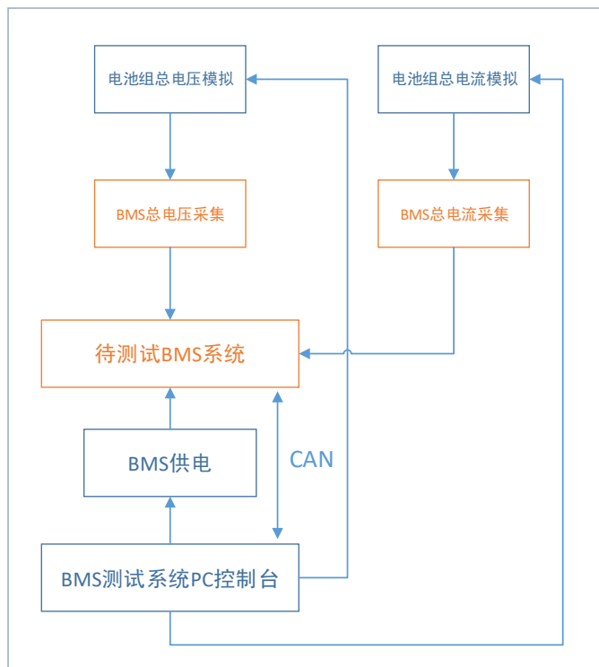
图3 电池总电压和总电流模拟与精度测试
