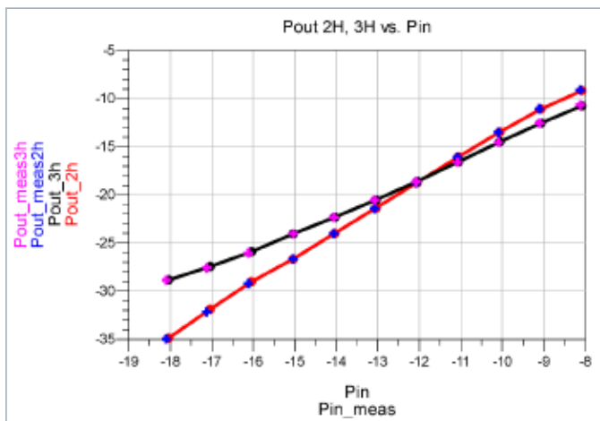
图6 Cardiff Model Lite模型仿真结果与实测结果比较
