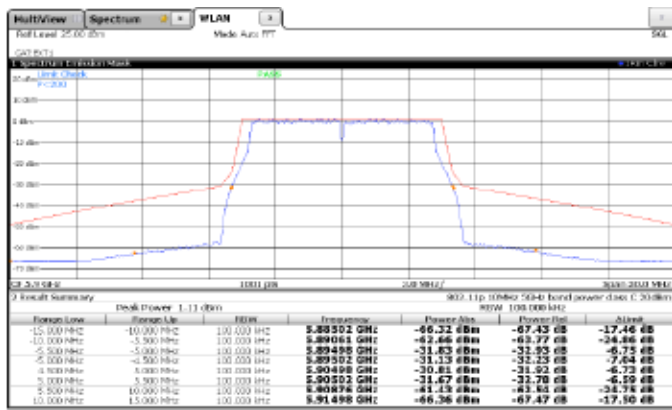
图29 DSRC/IEEE 802.11p频谱发射模板测试
