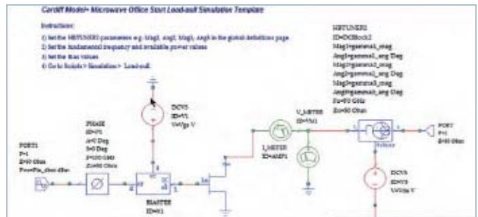
图5 在EDA软件中使用Cardiff 模型
