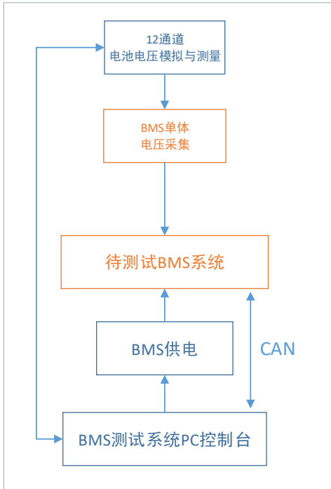
图4 电池单体电压模拟与精度测试
