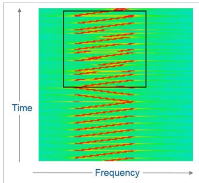
图2 由上升/下降斜率的多个脉冲构成的LoRa信号
