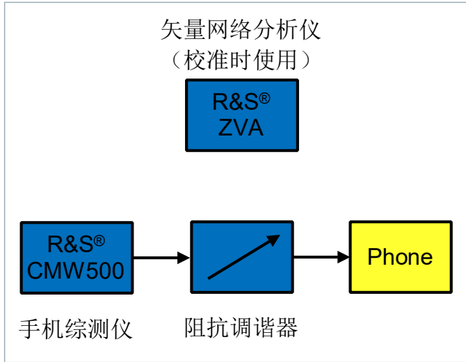
图9 手机终端负载牵引测量系统
