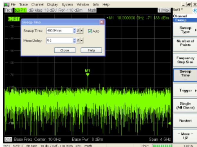
图13 ZVA对小信号的频谱分析结果和测试时间
