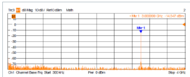
图12 ZVA的频谱分析结果
