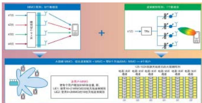
图1：大规模MIMO：波束赋形和空分复用组合
