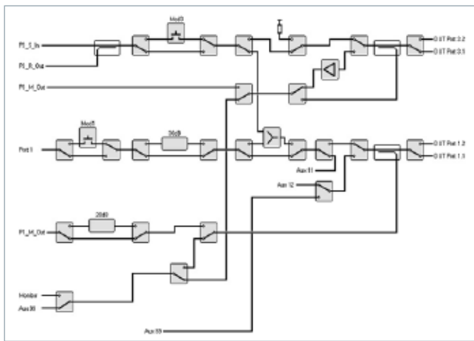
图15 OSP-TRM结构图
