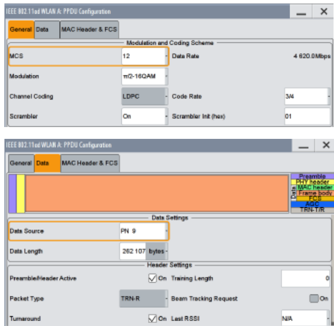
图4 SMW200A的11ad信号产生设置界面
