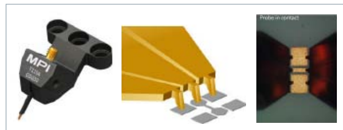
图5 典型GSG探针
