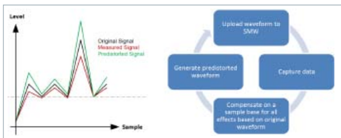
“直接”数字预失真方法的逐点补偿及迭代示意图
