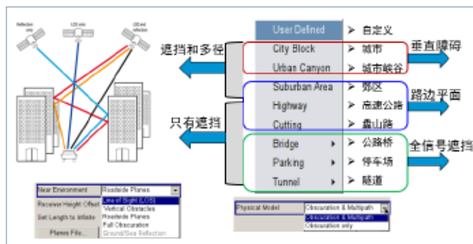
图20 遮挡效应及多径效应的模拟
