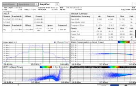
图a 数字预失真之前的功放测量结果
