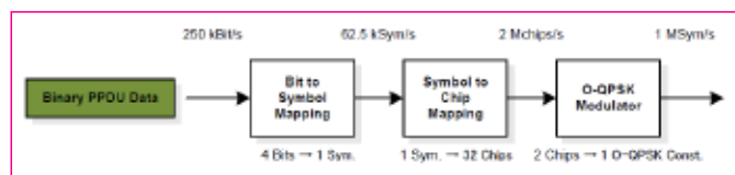
图3 O-QPSK PHY扩频和调制映射
