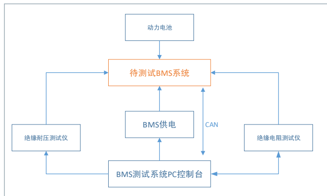
图8 BMS系统绝缘电阻、绝缘耐压测试
