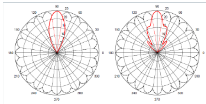
图9 采用角度扫描合成的等效全向辐射方向图(E、H面)
