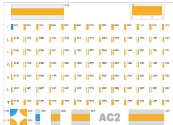
图6 典型GSG校准片
