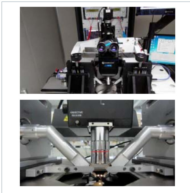
图5 在片负载牵引测量系统
