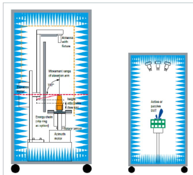
图15 暗室ATS1000的两种OTA测试场景
