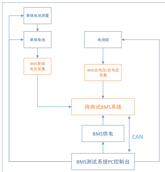
图12 电池充放电功能测试
