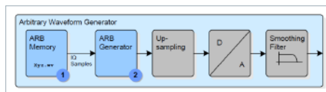
图7 ARB模式波形产生
