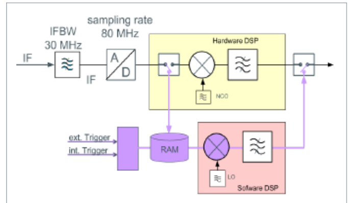
图8 ZVA脉冲时域参数测试硬件框图
