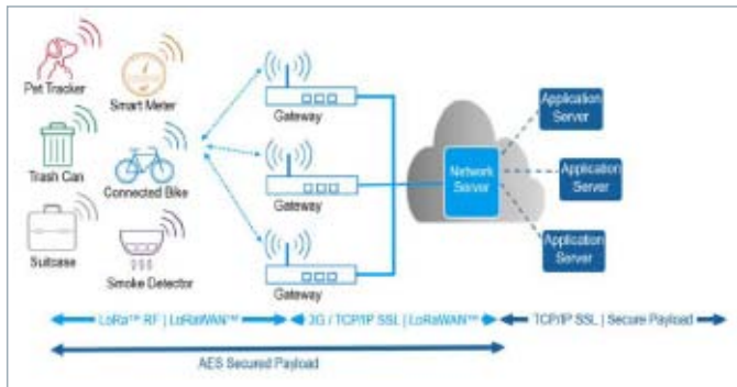
图4 LoRaWAN网络架构
