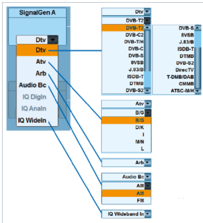
图5-3: R&S®BTC支持全球几乎广播电视标准
