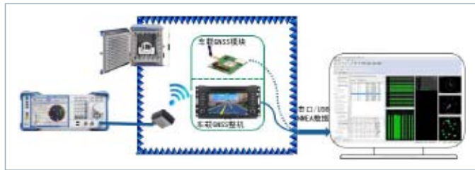
图56 车载导航接收机OTA测试框图
