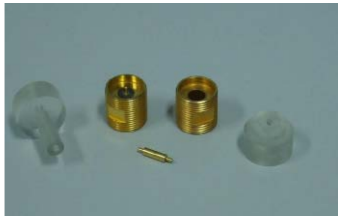
图9 同轴传输/反射法测量夹具
