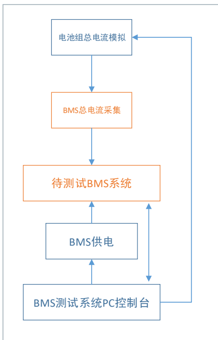
图7 电池SOC估算功能测试
