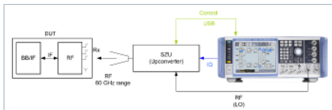
图13 终端接收指标测试
