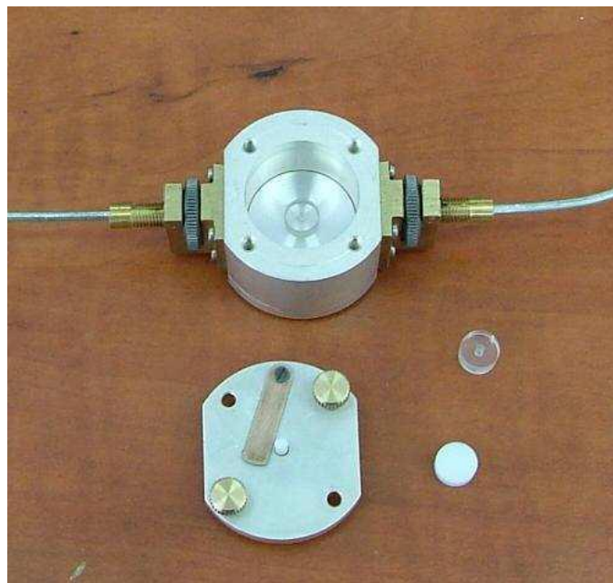
图4 微扰谐振腔
