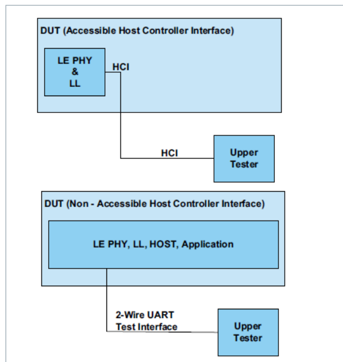
图2：direct test mode架构图
