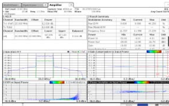
5b 经过一次数字预失真运算后的功放测量结果
