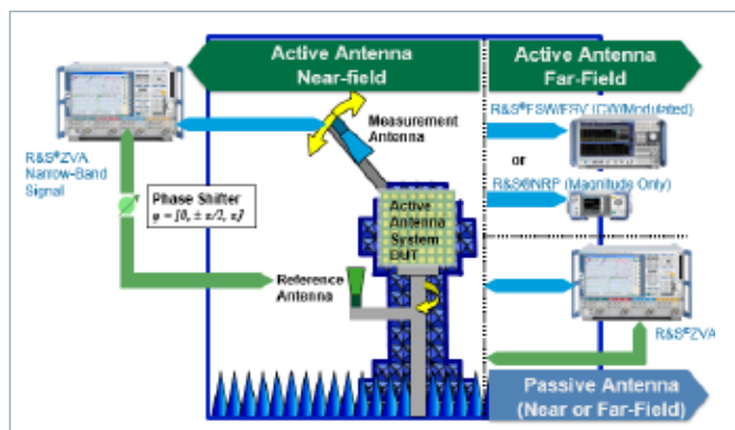
图2：OTA测试系统
