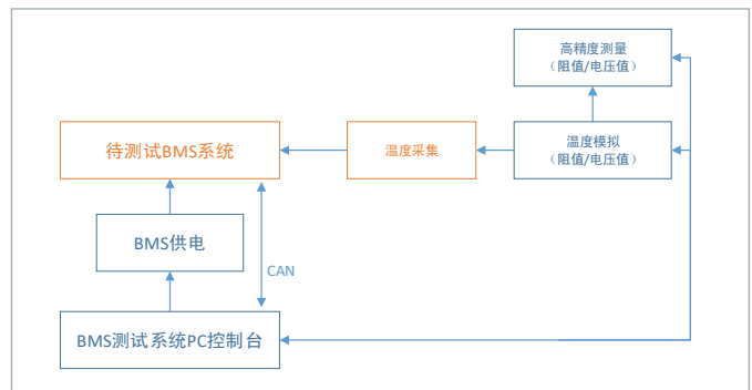
图6 电池组温度管理功能测试
