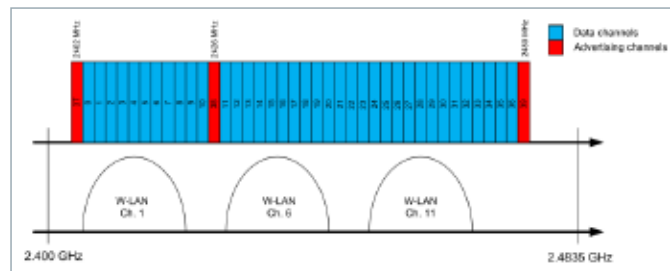
图25 Bluetooth无线通信频段划分
