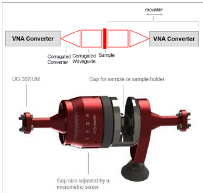
图8 波导传输/反射法测量薄膜材料夹具
