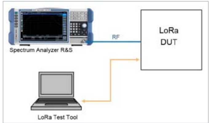
图6 LoRa发射机测试连接
