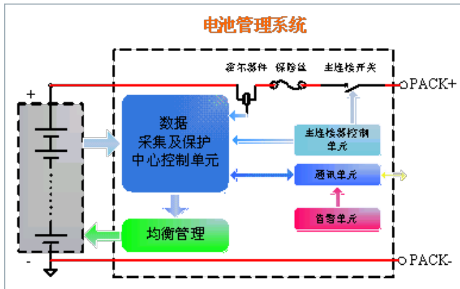
图1 BMS系统框图
