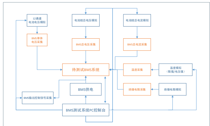
图6 电池组安全控制功能、故障诊断和处理功能测试
