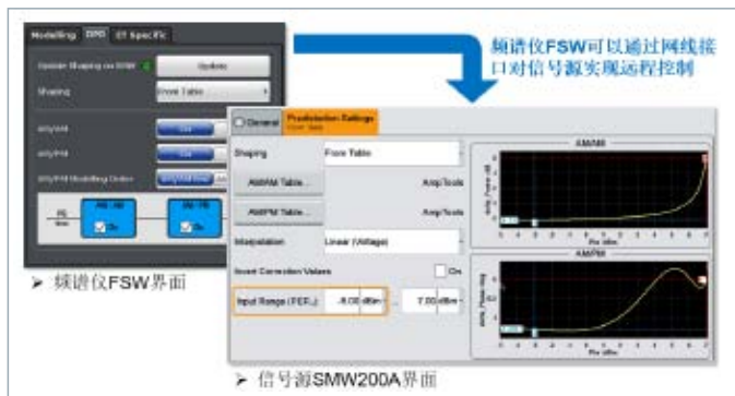
SMW200A和FSW数字预失真测试配置界面
