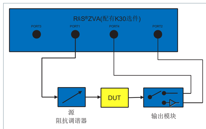
图8 基于ZVA矢量网络分析仪的噪声参数测量系统
