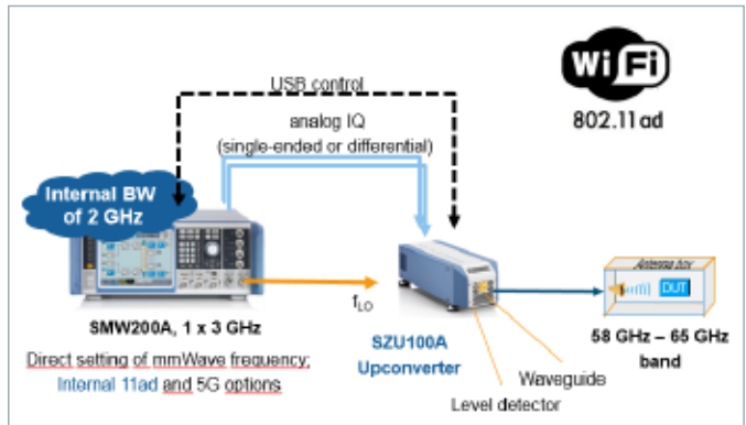
图11 SMW和SZU连接图
