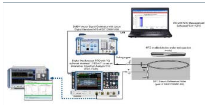
图70 车内NFC无线连接监听模式测试框图
