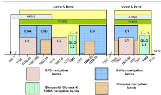
图2 GNSS卫星导航系统频段划分
