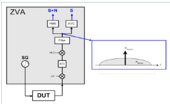
图4 ZVA-K30噪声系数测量原理
